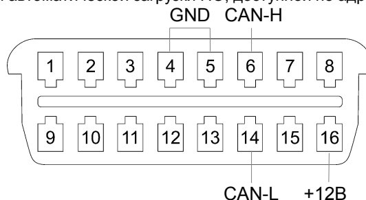
Рисунок 2. Подключение адаптера к разъему OBD-II.
